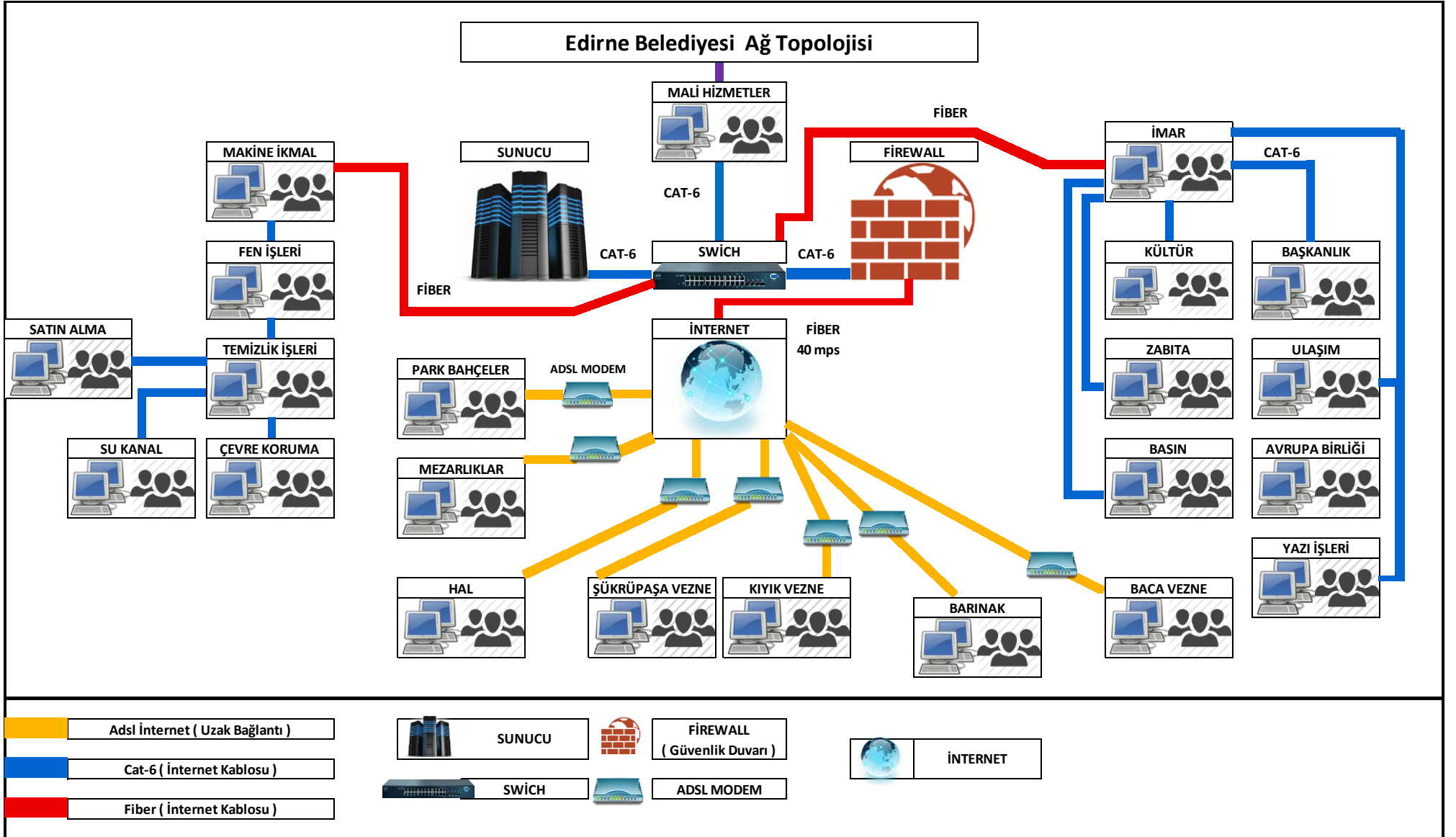
Belediyemize ait Ağ Yapı Şeması
